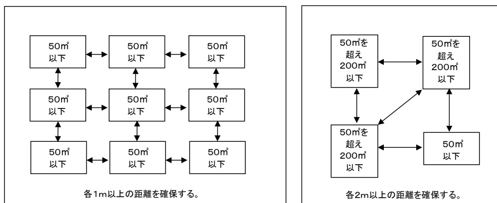
第3-4図 （1集積単位の面積は200㎡以下とする。）
