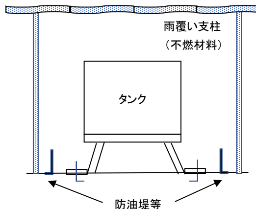
第2-24図 雨覆いを設けた例
