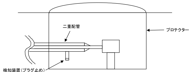
第2-7図 地下埋設配管を二重配管とし、検知管を設ける方法
