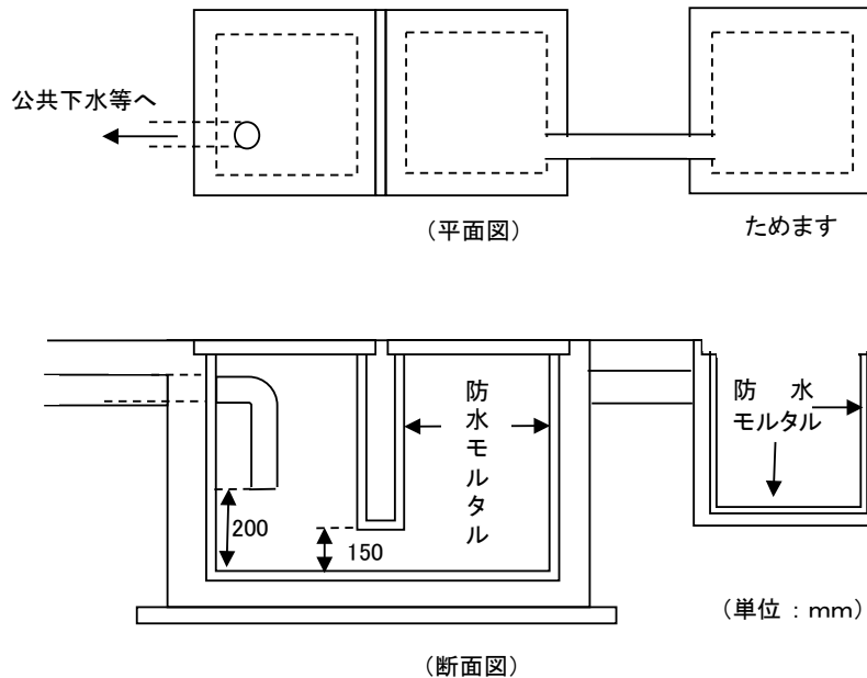
第 2 - 1 1 図 ためます及び油分離槽を別々とした例
