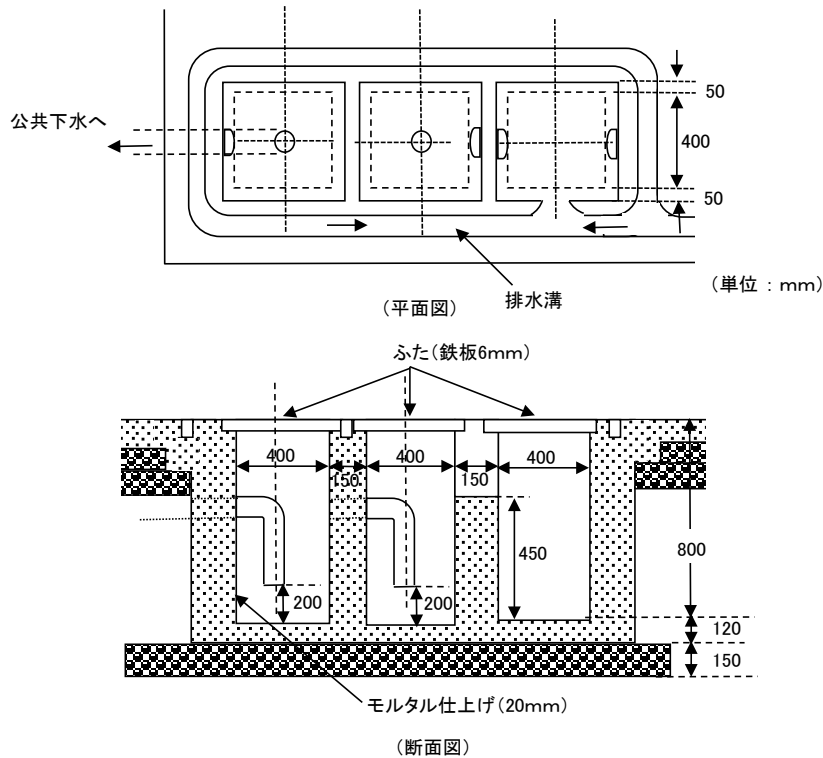
第 2 - 1 2 図 油分離槽の例
