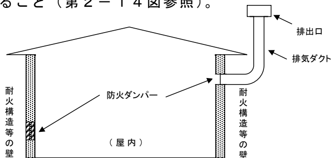
第2-14図 防火ダンパーの設置例
