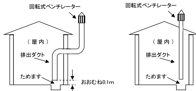
第2-16図 強制排出設備の例
