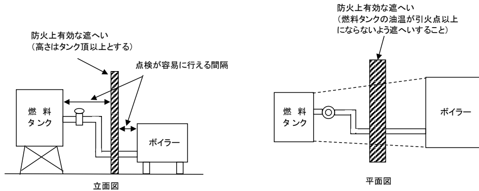
第2-17図 防火上有効な遮へいを設ける例
