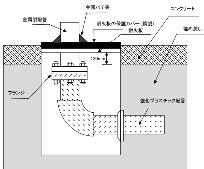
第 2 - 6 図 地下ピット内での接続例その 2
