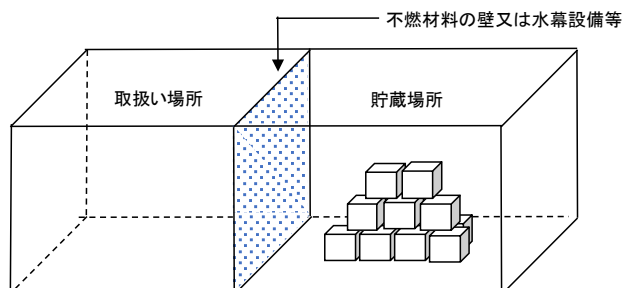
第3-5図 合成樹脂類の取扱場所と貯蔵場所を区画する例
