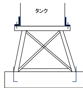
第2-19図 架台上に固定する例
