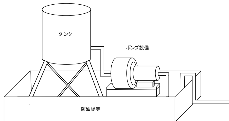
第2-23図 ポンプ設備を防油堤等内に設ける例
