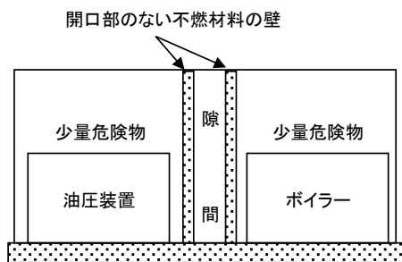
第1-7図 認められない例
