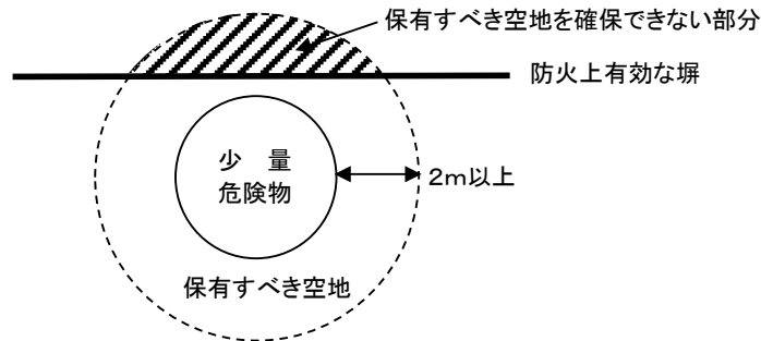
第2-8図 塀を設ける場合の遮へい範囲
