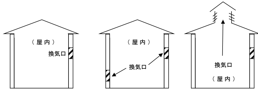
第2-13図 自然換気設備の例
