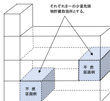
第 1 - 1 5 図 新築工事中的場合 第 1 - 1 6 図 不燃区画例による場合
