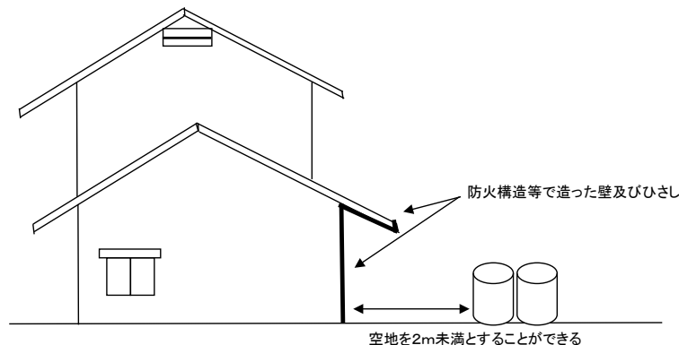
第2-9図 壁を設ける場合の高さ
