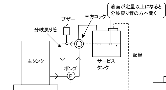
第2-1図 分岐装置
