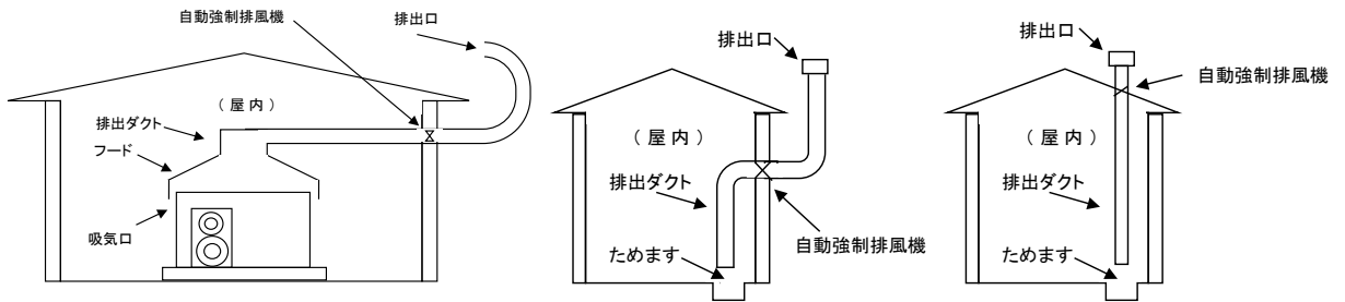
第2-15図 自動強制排出設備の例
