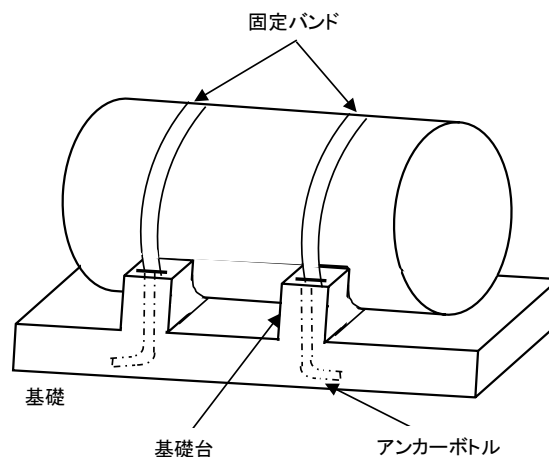
第2-20図 タンクを直接基礎に固定しない例
