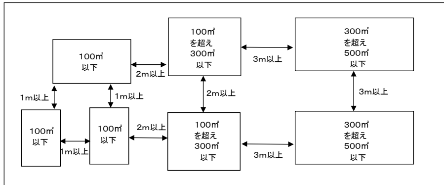
第3-5図 (1集積単位の面積は500㎡以下とする。)
