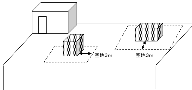
第 1 - 1 4 図 保有空地例により複数設置する場合
