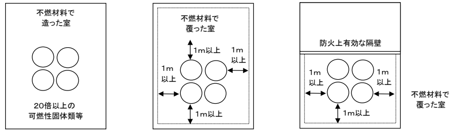
第 3 - 3 図 20 倍以上の可燃性固体類等を屋内に貯蔵し、又は取り扱う場合の例
