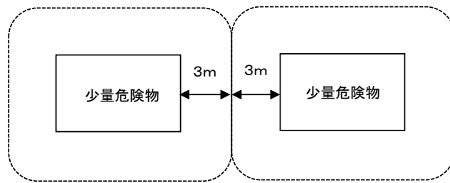
第1-9図 保有空地例により複数設置する場合
