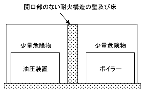
第1-8図 認められる例
