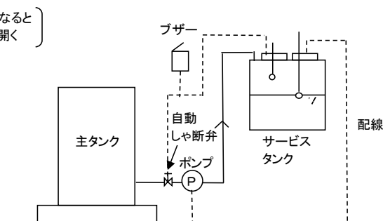
第2-2図 二重フロートスイッチによるしゃ断弁
