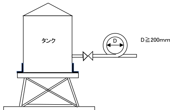
第2-22図 可撓管継手を設けることができない場合の例
