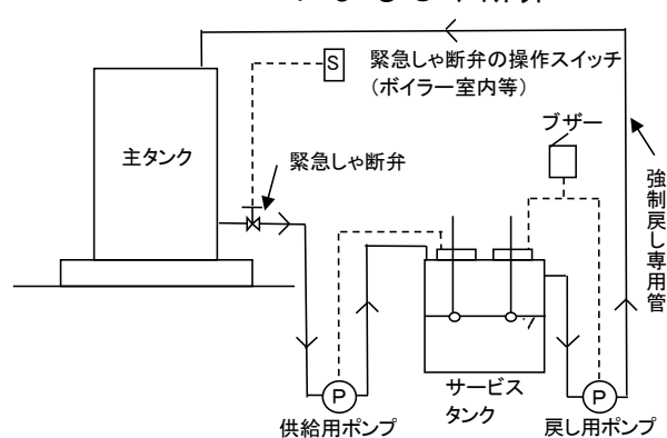
第2-4図 強制戻し専用管及び緊急しゃ断弁
