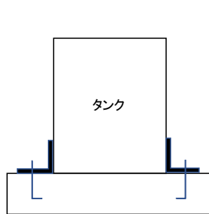
第2-18図 基礎上に固定する例
