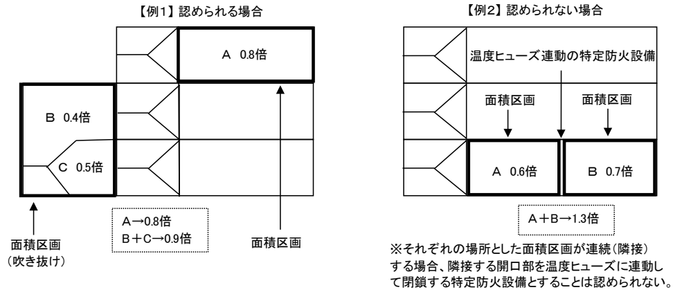
第1-11図 面積区画による場合
