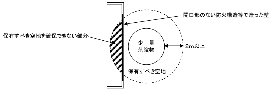
第 2 - 1 0 図 壁を設ける場合の遮へい範囲
